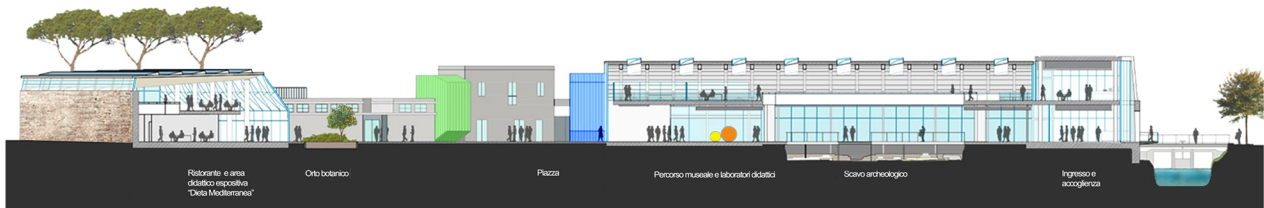
Sezione longitudinale
